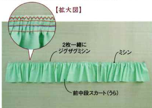
8. 下糸を引き、つけ寸法までギャザー寄せて、切り替え線をミシンで縫う。縫い代はジグザグミシンで始末する。
