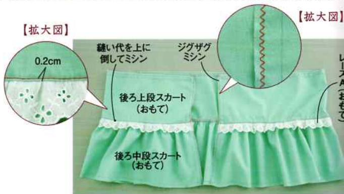
9. 縫い代を上倒して、おもて側からミシンで縫う。後ろ中心線をジグザグミシンで始末する。
