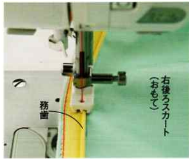
9. 右ファスナーの務歯を押え金の右の溝にはめ、上から下の方向に縫い、縫えるところまで縫って返し縫いをする。
