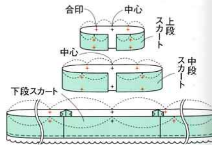
6. 上図の様にスカートをそれぞれ8等分して、印をつける。
