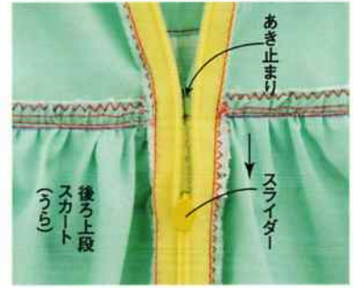
7. スライダーをあき止まりより下げる。
