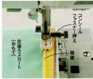
8. ミシンの押え金をコンシールファスナー押えに替える。左ファスナーの務歯を押え金の左の溝にはめ、上から下の方向に縫い、縫えるところまで縫って返し縫いをする。
