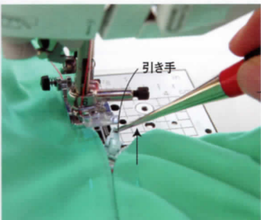
8. 引き手の厚みで縫いにくくなったら、目打ちを使って引き手を上までスライドする
