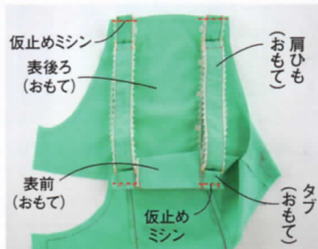
3. タブを表前身頃につけ、肩ひもを表後ろ身頃につける
